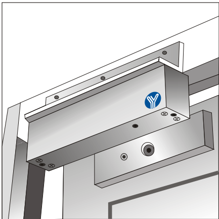
1. 安裝效果圖
