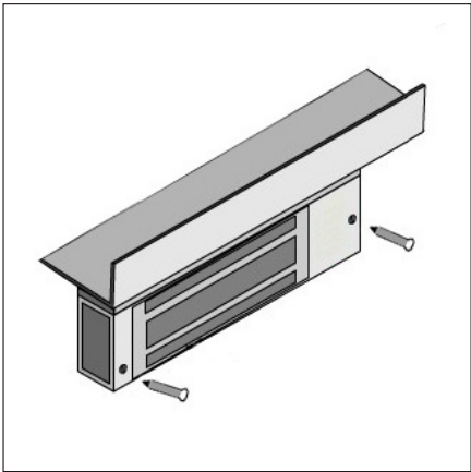
6. 擰緊磁力鎖并且測試
