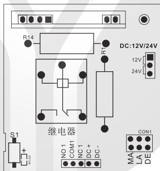
控制器主板簡化圖：
