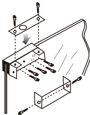
电插锁支架安装效果
