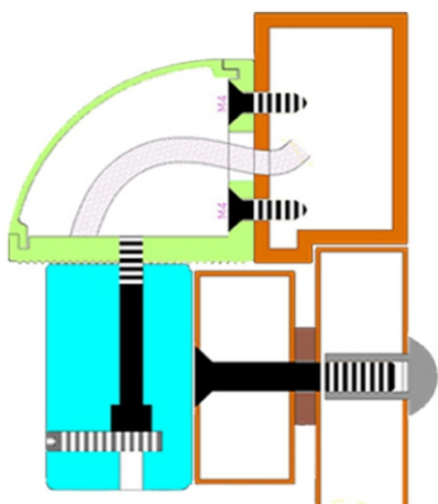
LC型支架電源線內藏， 美觀及防止破壞線路。
