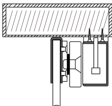
搭配U型輔助架安裝在無框玻璃門
