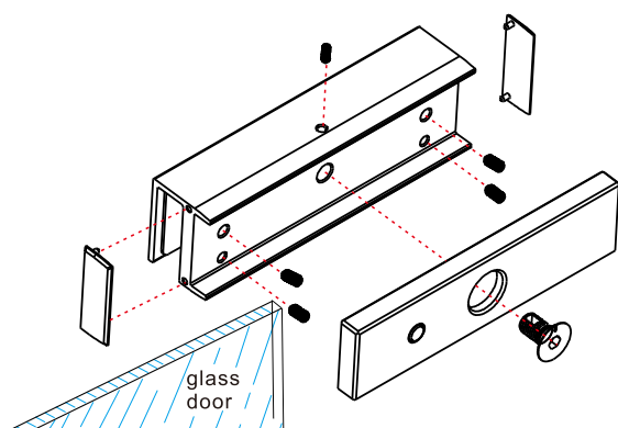
U型支架安裝效果
