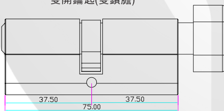
單開鑰匙帶旋鈕開門(標準出廠配套)
