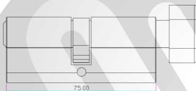
單開鑰匙帶旋鈕開門(標準出廠配套)
