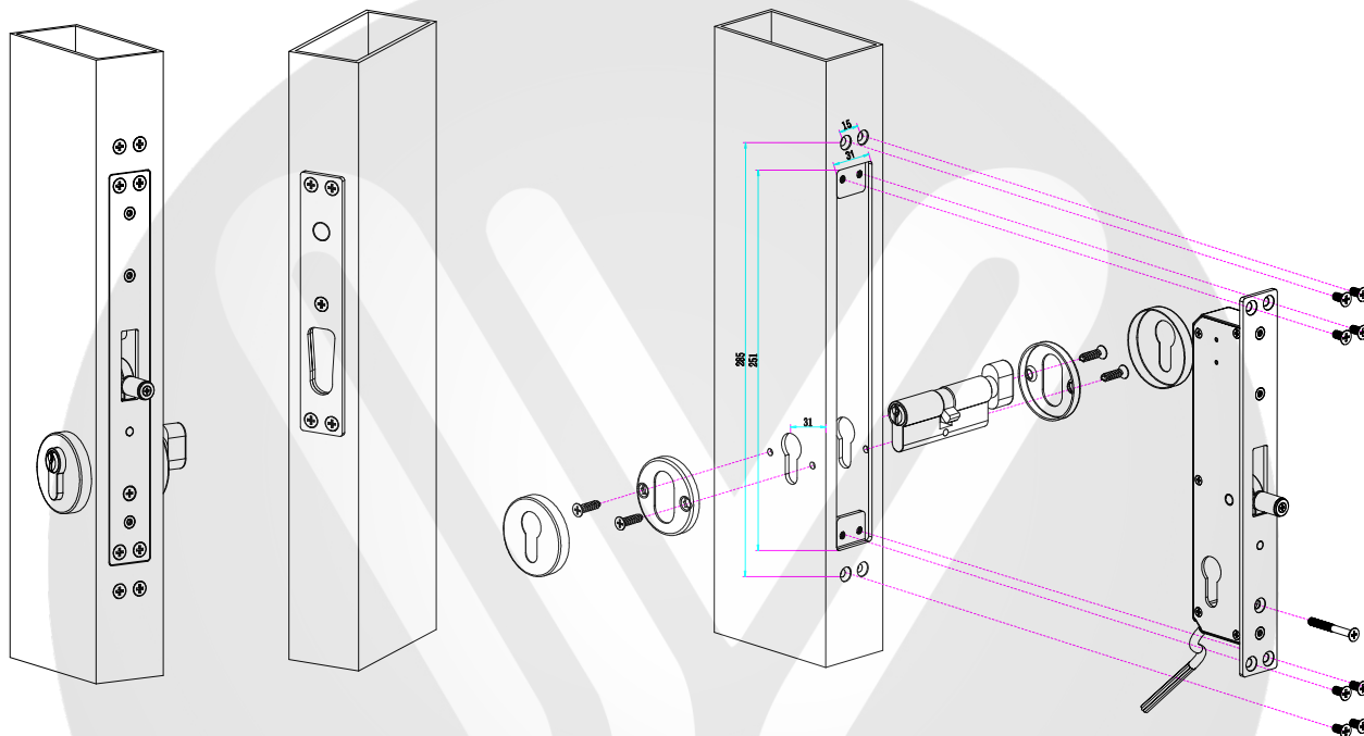
空心門開孔圖
