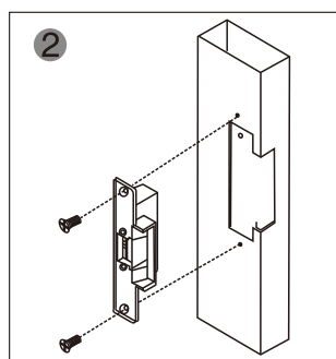
將電鎖口安裝在切割好的位置，接上電源，并且進行測試。
