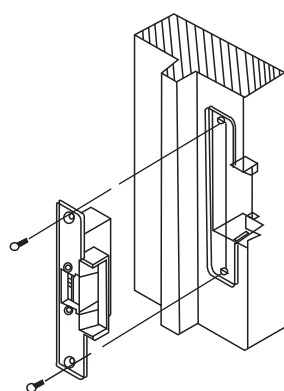
木質門框
