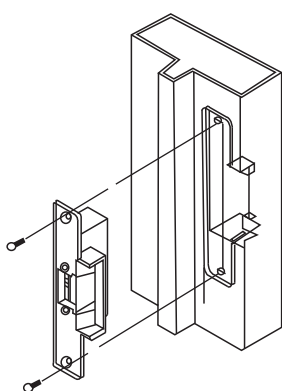
金屬門框
