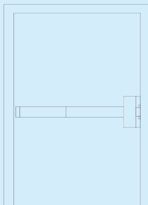
單開門安裝：橫式鎖
