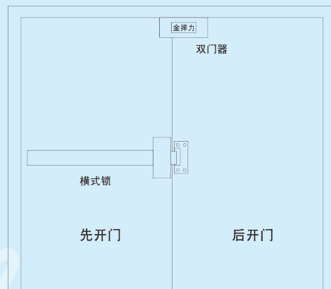
雙開門安裝：橫式鎖+雙門器
