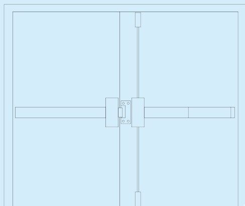
雙開門安裝：橫式鎖+天地栓鎖
