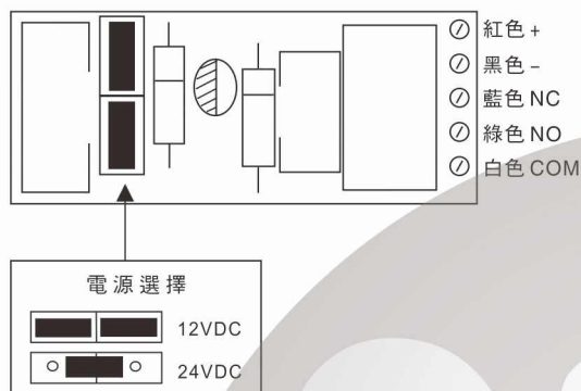
YM-180M-S, YM-280M-S, YM-500M-S綫路板圖
