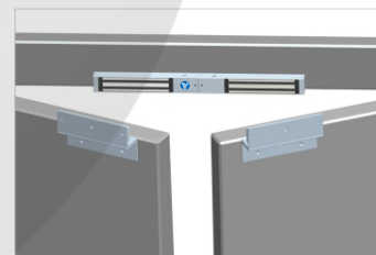
ZL型辅助支架
