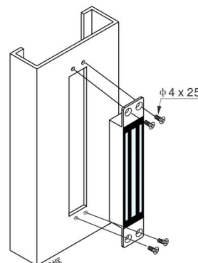
固定螺絲
