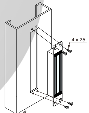
固定螺絲
