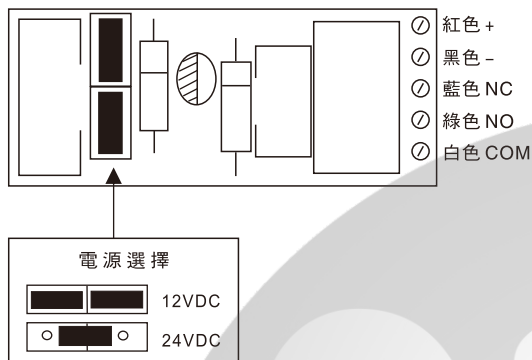
YM-180M-S, YM-280M-S, YM-500M-S綫路板圖
