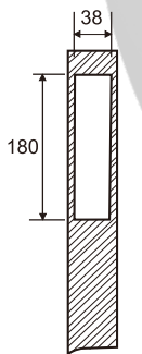
挖空尺寸
