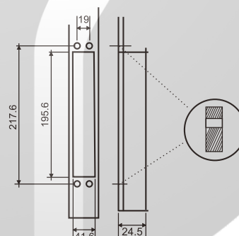
挖空尺寸
